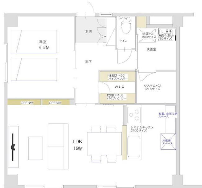
【間取り図】
