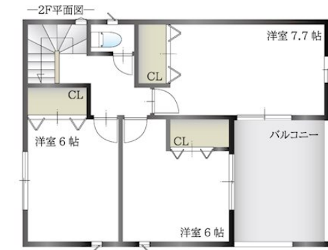
【間取り図】
